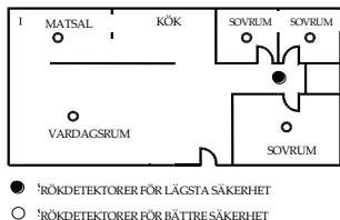
Figur 1: Monteringsplatser för rök- och värmedetektorer i lägenheter eller enfamiljshus med bara ett sovrum
