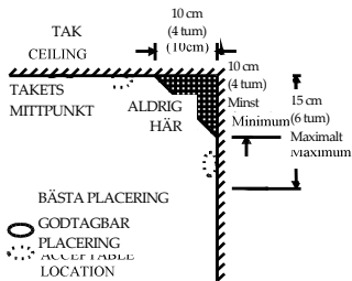
Figur 3: Rekommendationer för bästa och godtagbara monteringsplatser vid montering av rök- och värmedetektorer.
